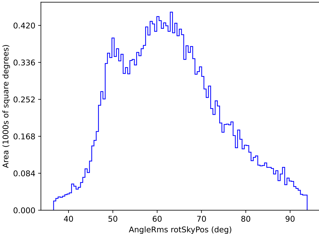
roman_v3.3_10yrs All sky y band: AngleRms rotSkyPos
