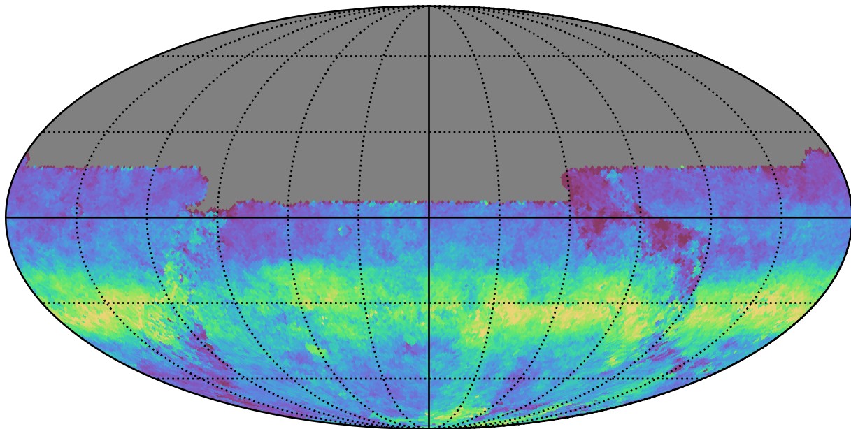
roman_v3.3_10yrs All sky u band: AngleRms rotSkyPos
