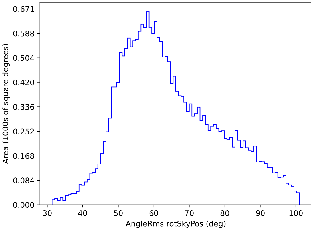
roman_v3.3_10yrs All sky u band: AngleRms rotSkyPos
