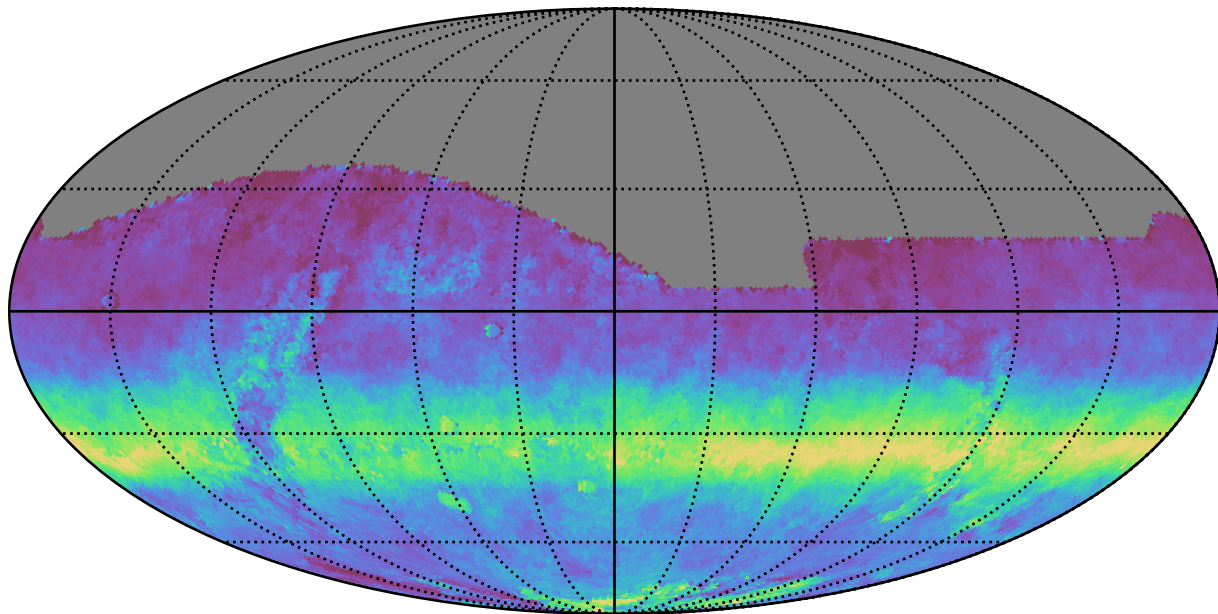
roman_v3.3_10yrs All sky r band: AngleRms rotSkyPos
