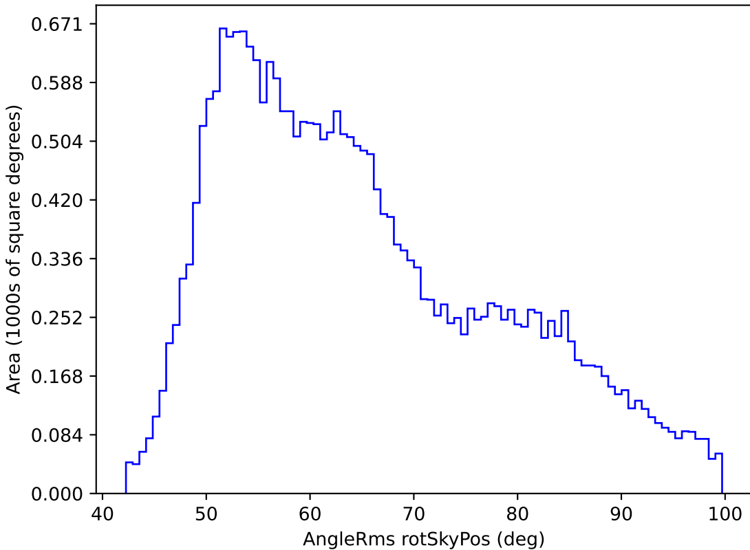
roman_v3.3_10yrs All sky r band: AngleRms rotSkyPos
