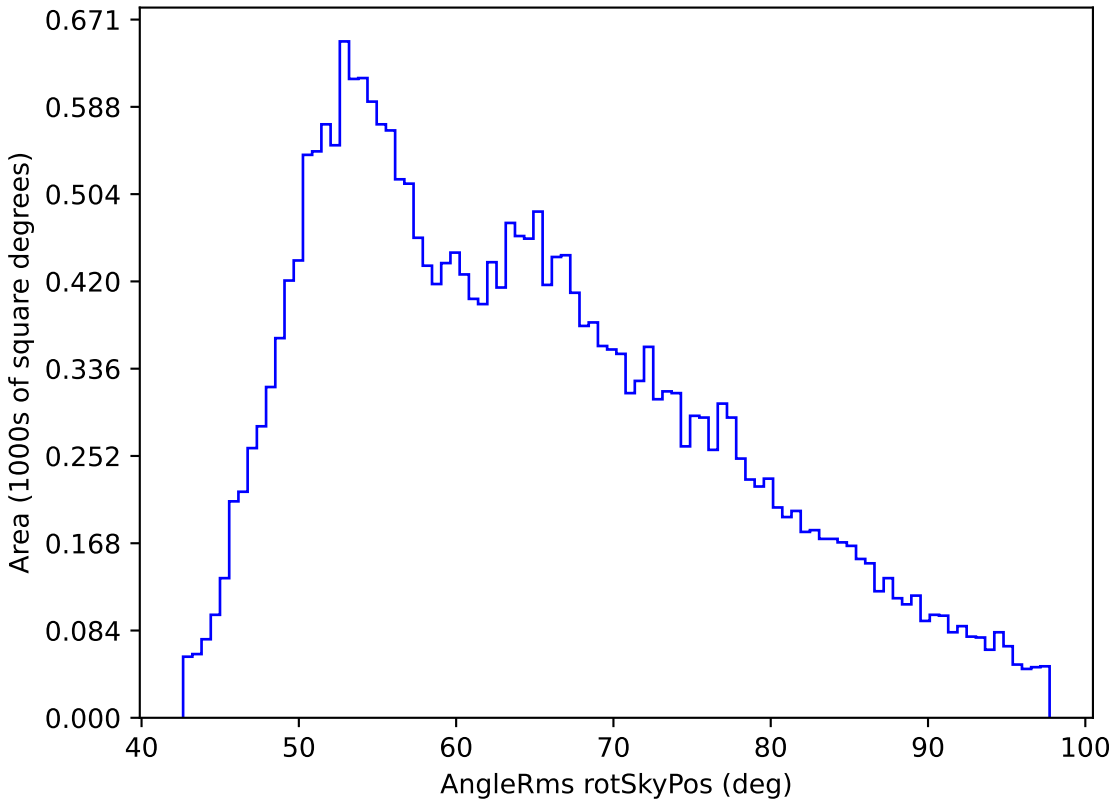
roman_v3.3_10yrs All sky i band: AngleRms rotSkyPos
