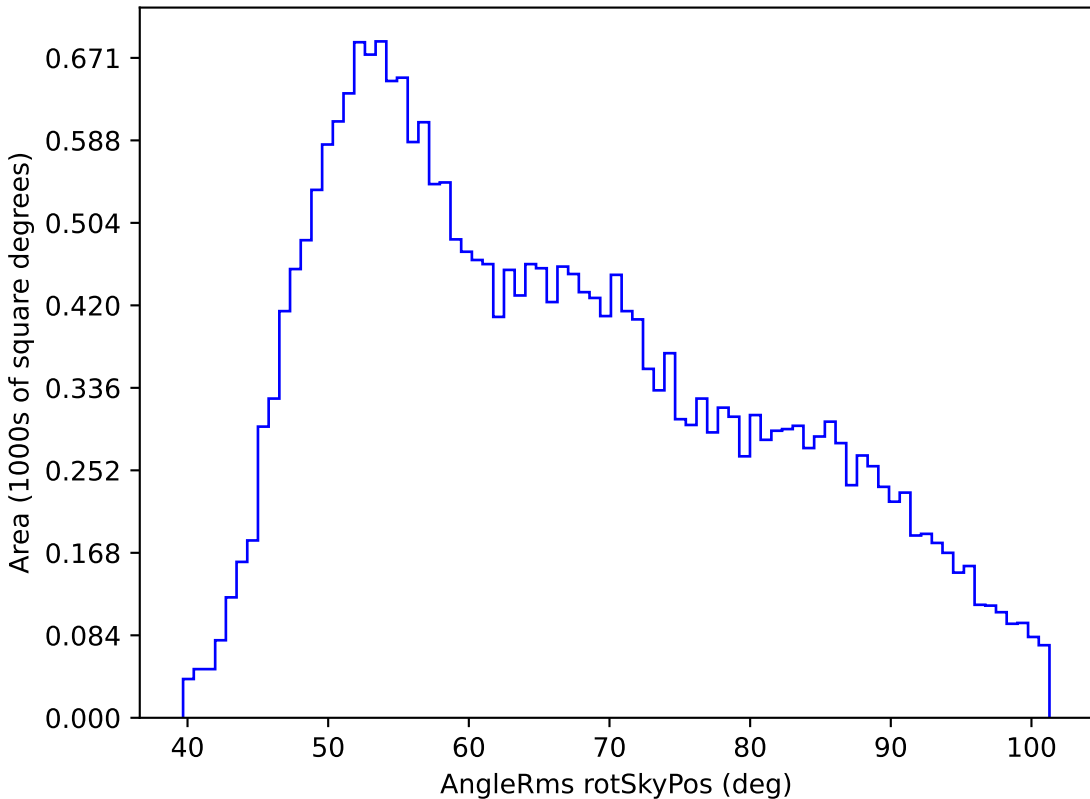
roman_v3.3_10yrs All sky g band: AngleRms rotSkyPos
