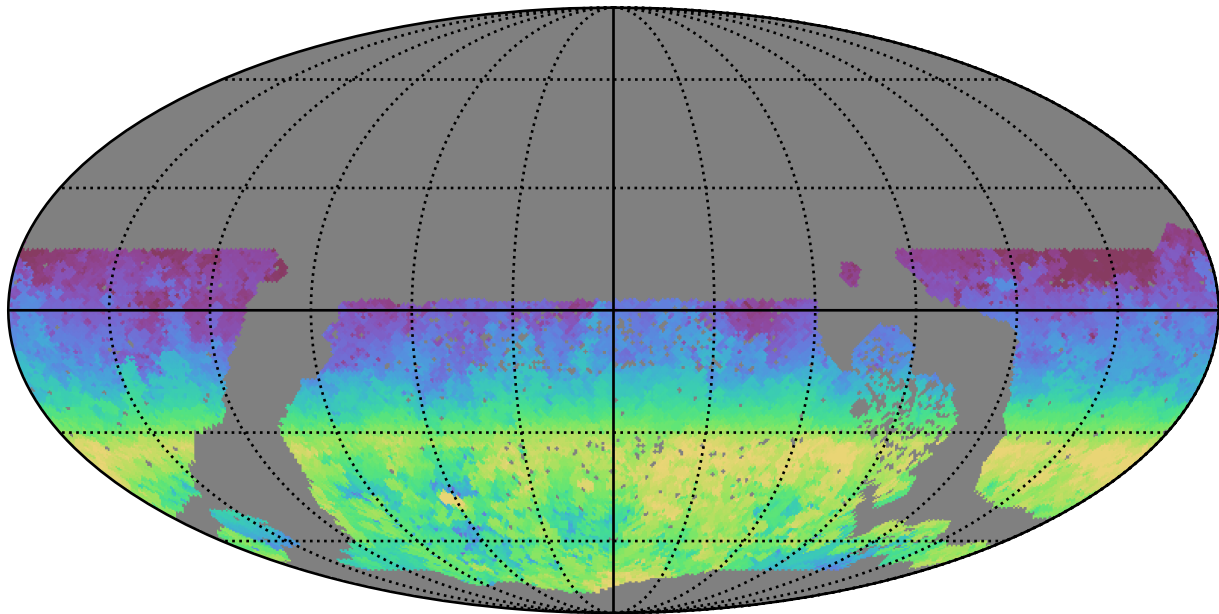
roman_v3.3_10yrs WFD z band: AngleRange rotSkyPos
