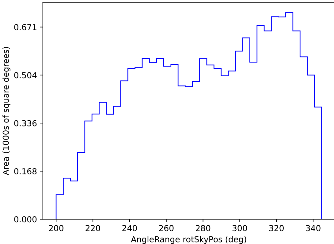
roman_v3.3_10yrs WFD z band: AngleRange rotSkyPos
