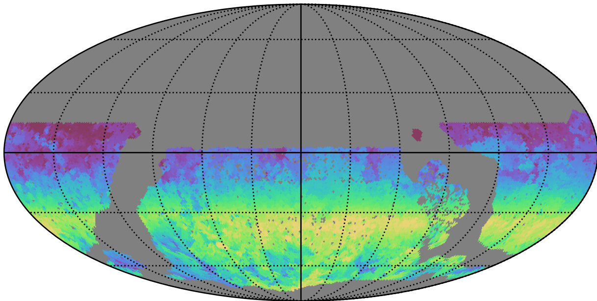
roman_v3.3_10yrs WFD y band: AngleRange rotSkyPos
