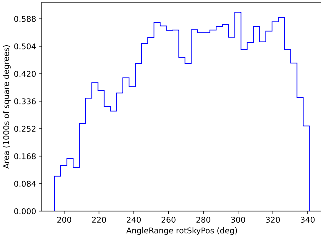
roman_v3.3_10yrs WFD y band: AngleRange rotSkyPos
