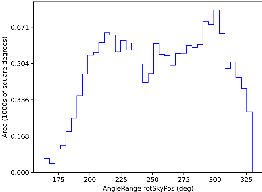
roman_v3.3_10yrs WFD u band: AngleRange rotSkyPos
