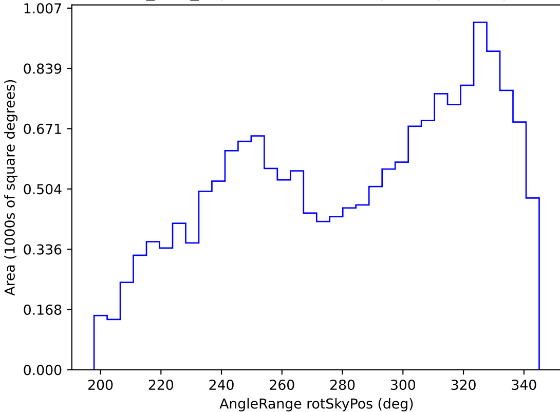
roman_v3.3_10yrs WFD i band: AngleRange rotSkyPos
