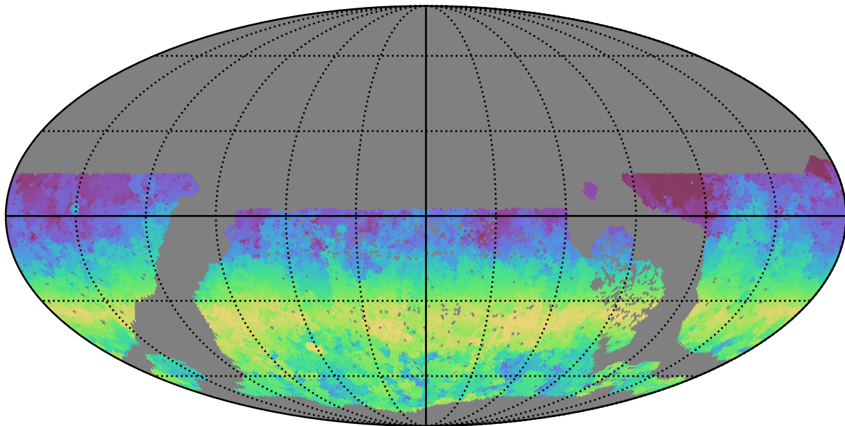
roman_v3.3_10yrs WFD g band: AngleRange rotSkyPos
