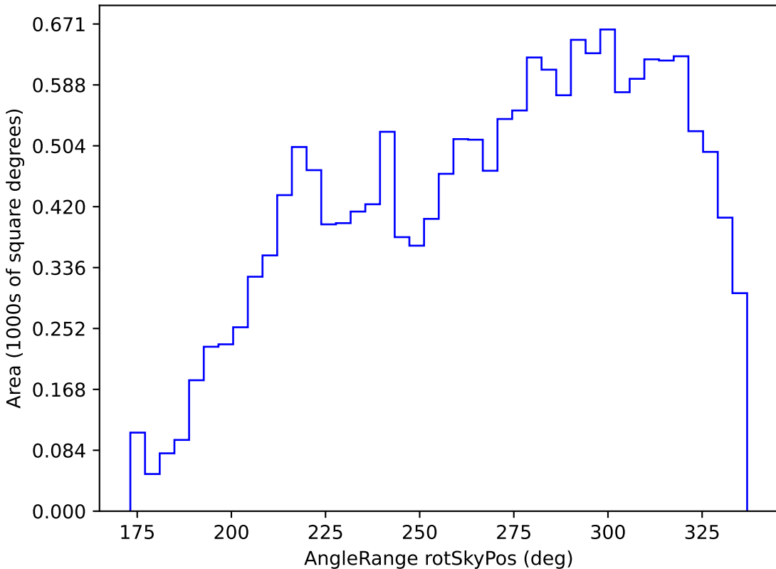
roman_v3.3_10yrs WFD g band: AngleRange rotSkyPos
