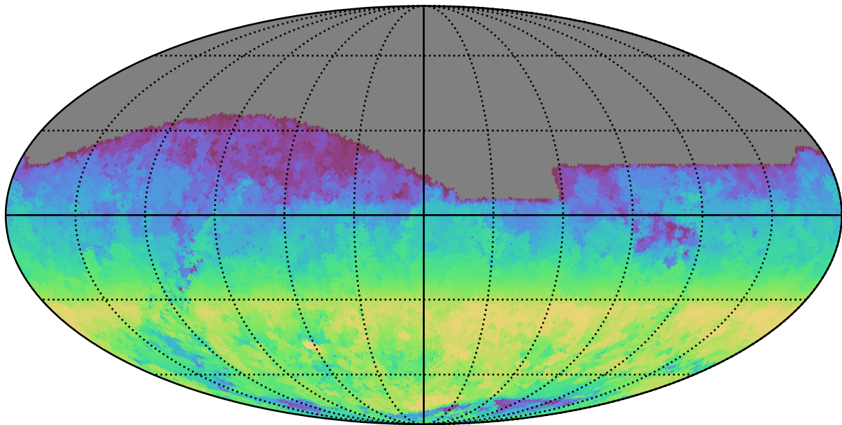
roman_v3.3_10yrs All sky z band: AngleRange rotSkyPos
