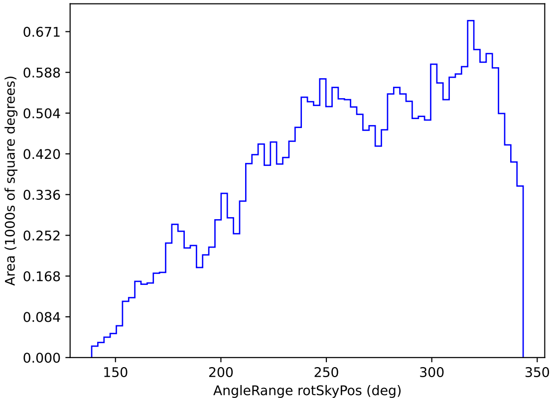
roman_v3.3_10yrs All sky z band: AngleRange rotSkyPos
