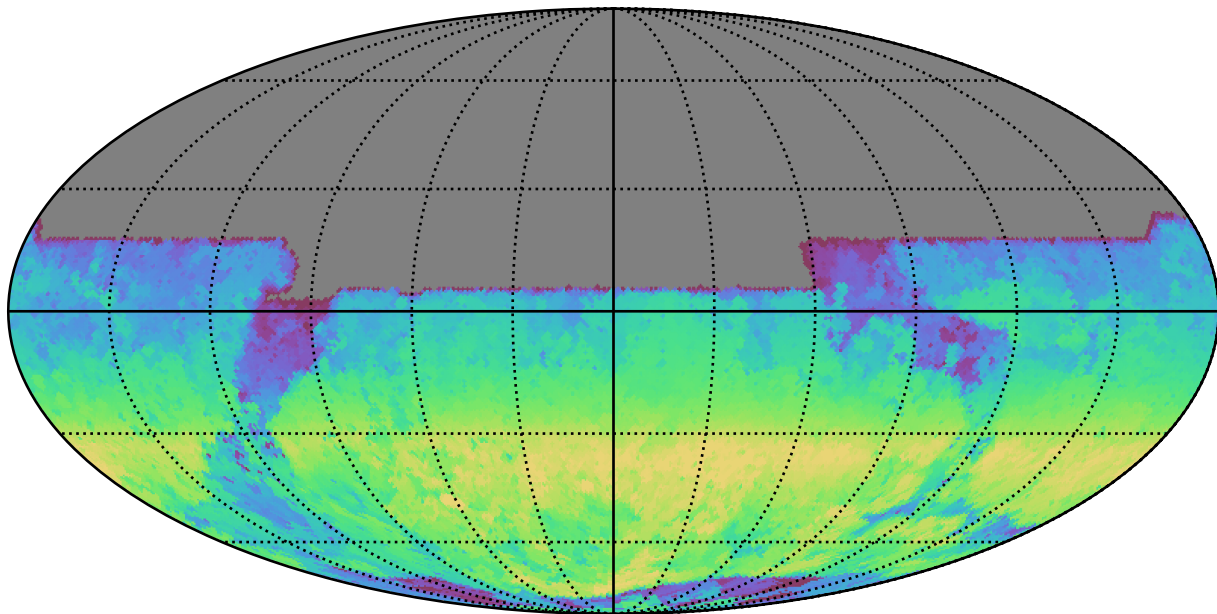
roman_v3.3_10yrs All sky y band: AngleRange rotSkyPos
