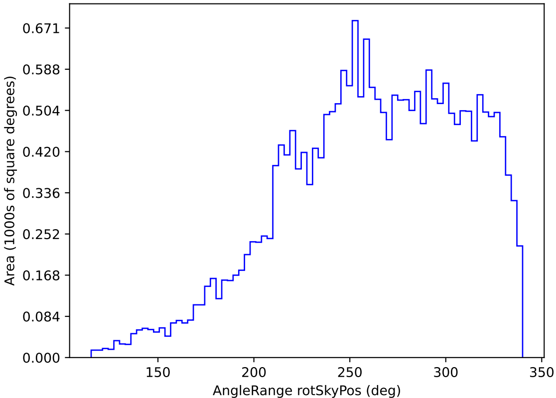
roman_v3.3_10yrs All sky y band: AngleRange rotSkyPos
