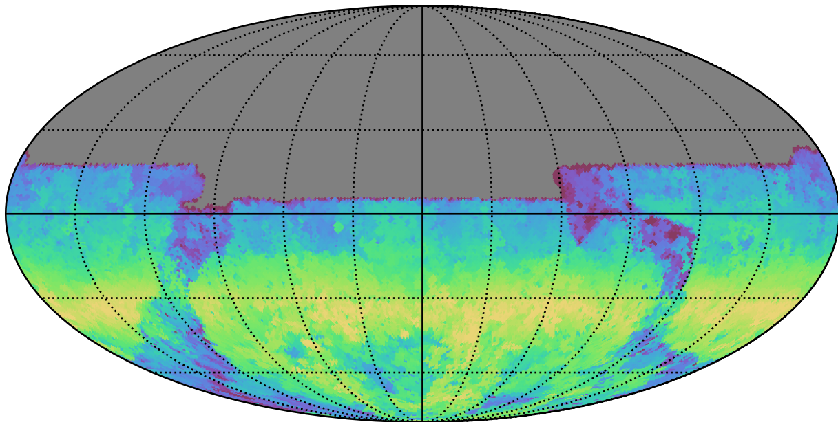
roman_v3.3_10yrs All sky u band: AngleRange rotSkyPos
