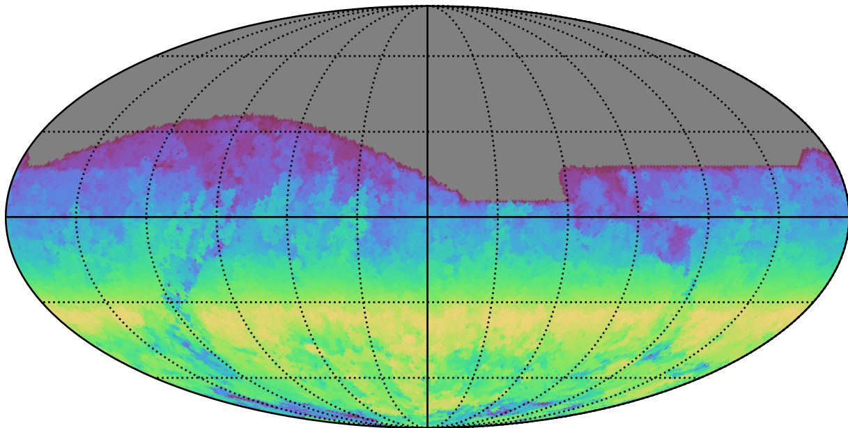
roman_v3.3_10yrs All sky r band: AngleRange rotSkyPos
