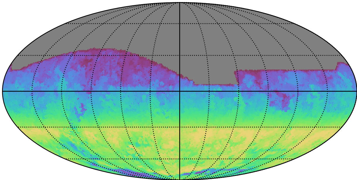
roman_v3.3_10yrs All sky i band: AngleRange rotSkyPos
