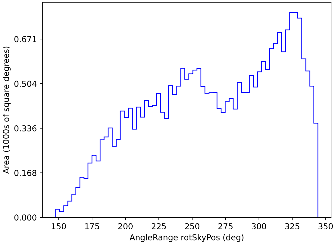
roman_v3.3_10yrs All sky i band: AngleRange rotSkyPos
