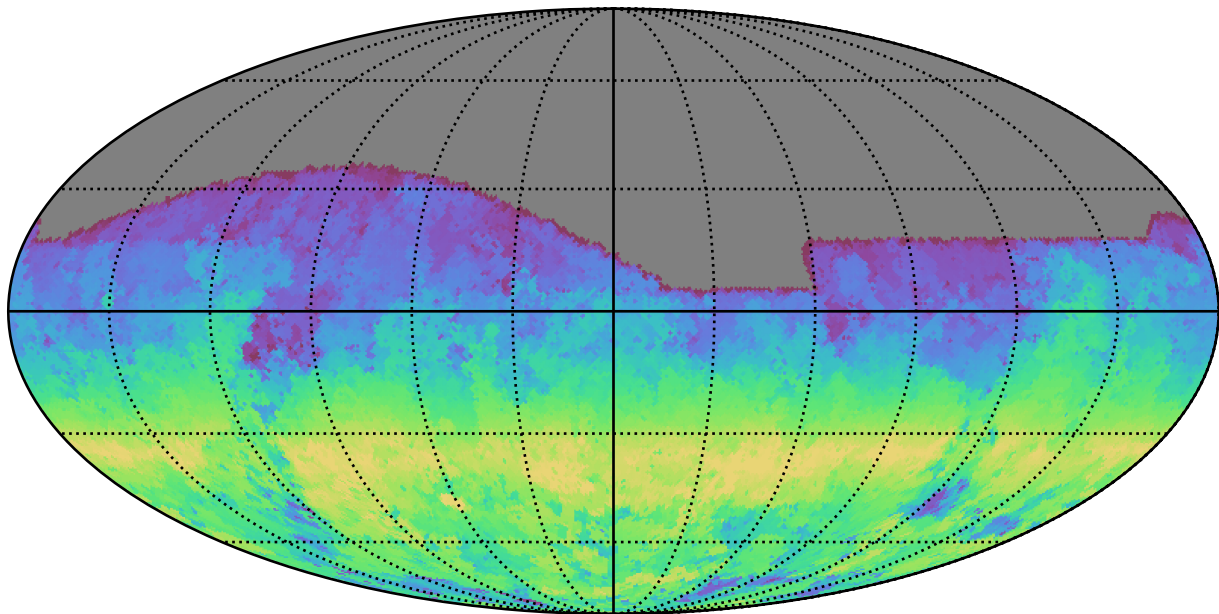
roman_v3.3_10yrs All sky g band: AngleRange rotSkyPos
