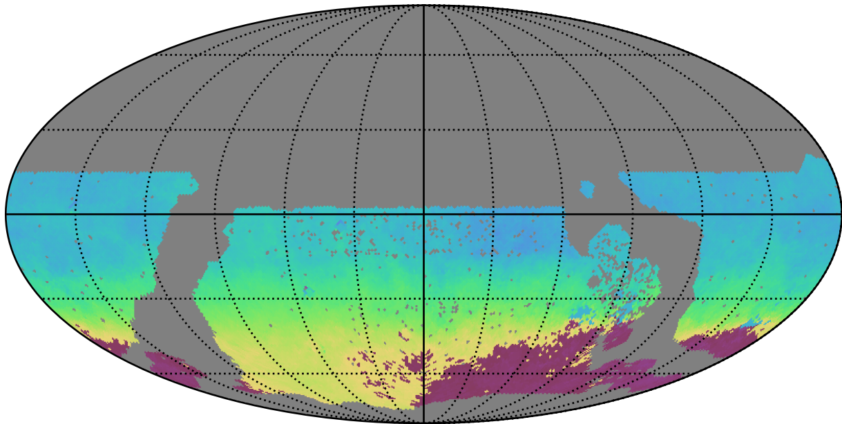
roman_v3.3_10yrs WFD z band: AngleMean rotSkyPos
