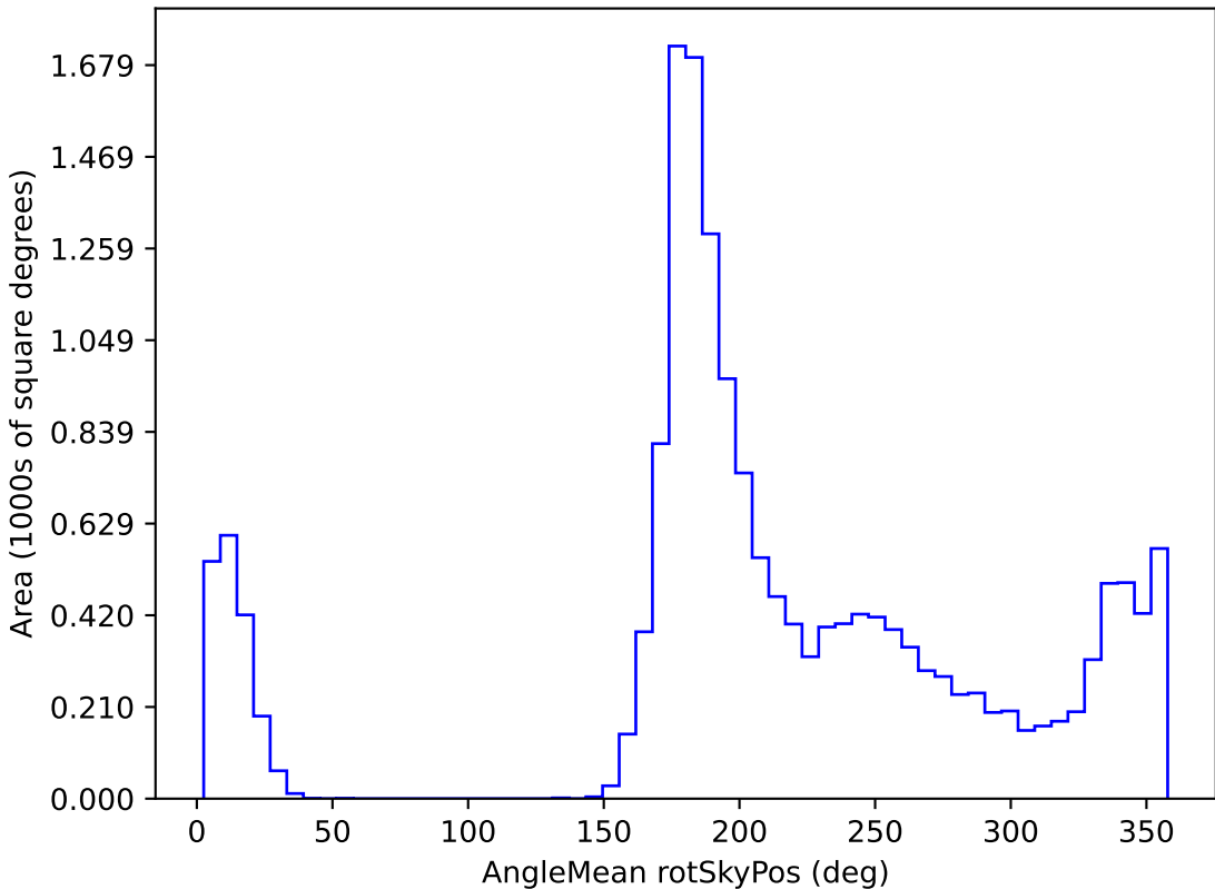
roman_v3.3_10yrs WFD z band: AngleMean rotSkyPos
