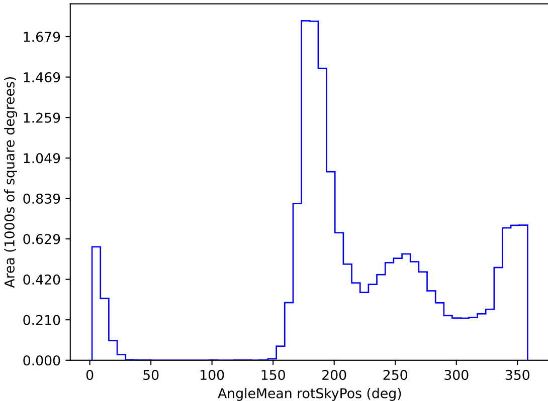
roman_v3.3_10yrs WFD y band: AngleMean rotSkyPos
