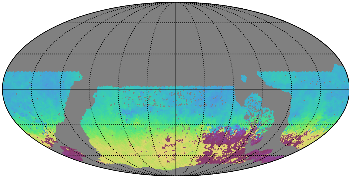
roman_v3.3_10yrs WFD u band: AngleMean rotSkyPos
