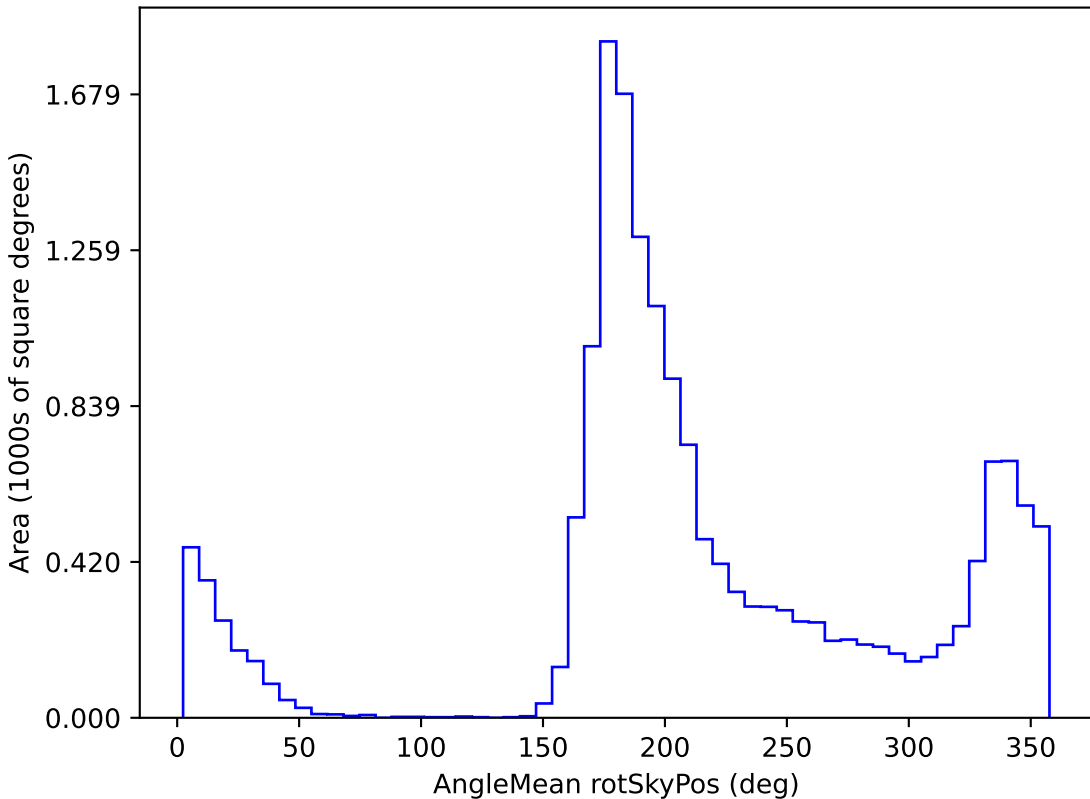
roman_v3.3_10yrs WFD u band: AngleMean rotSkyPos
