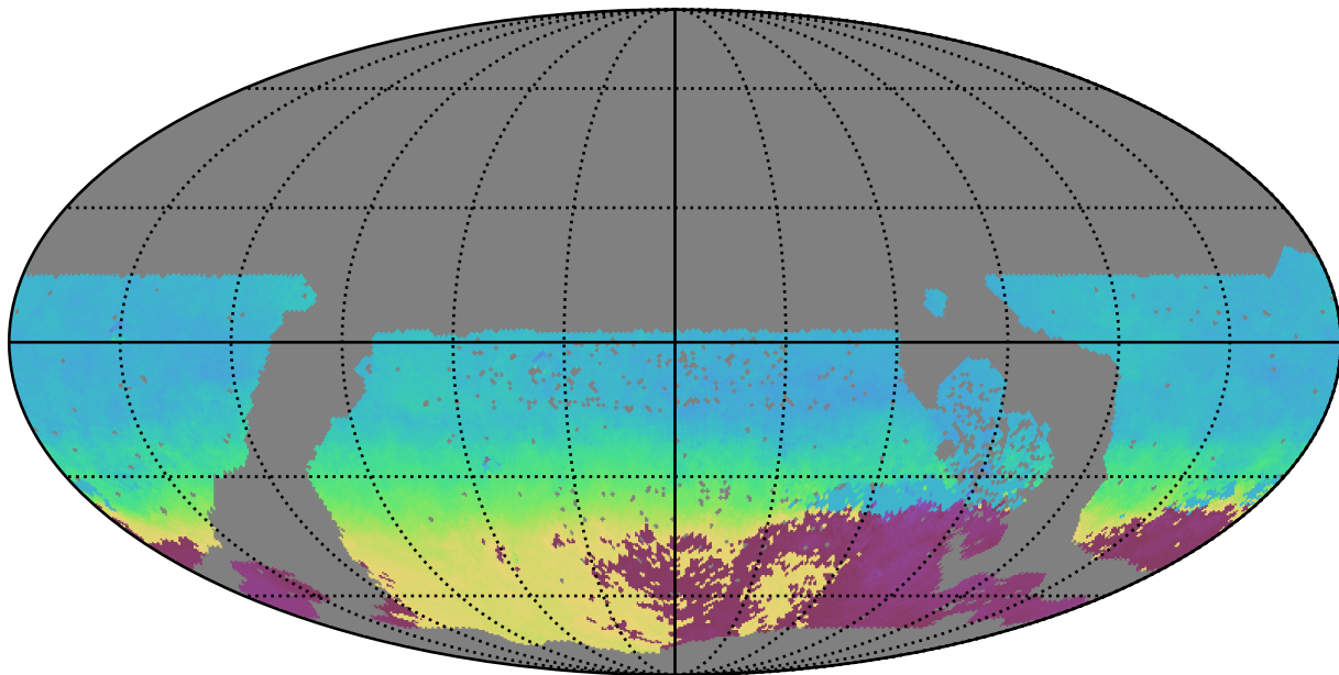
roman_v3.3_10yrs WFD r band: AngleMean rotSkyPos
