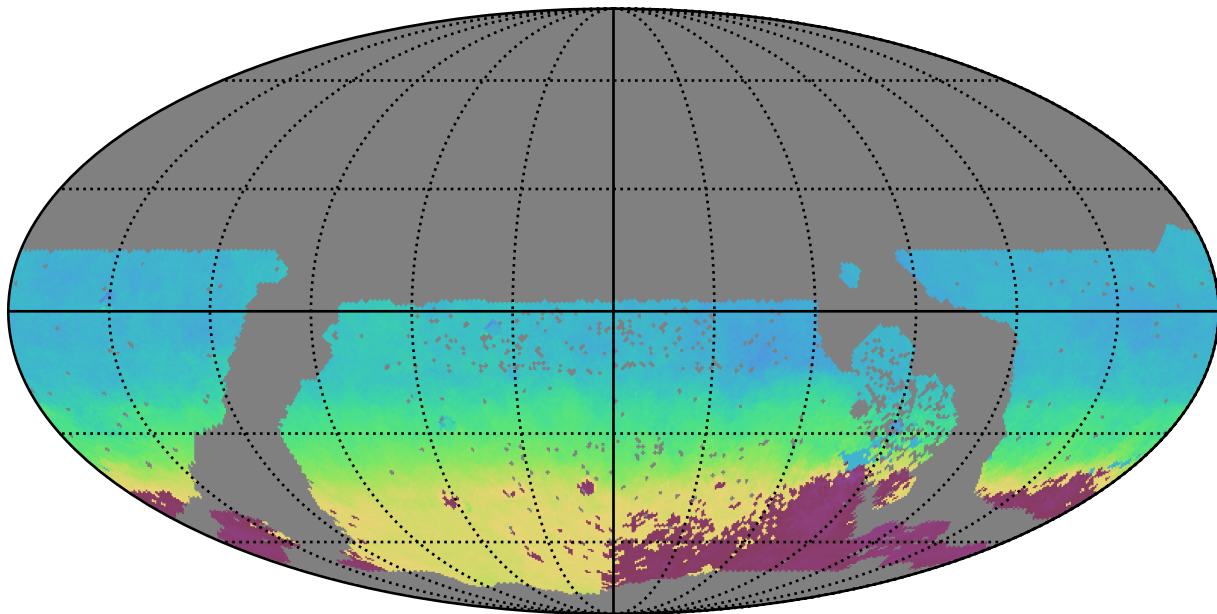
roman_v3.3_10yrs WFD i band: AngleMean rotSkyPos
