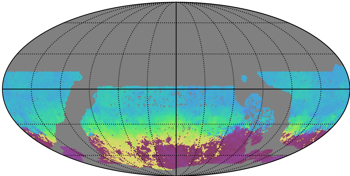
roman_v3.3_10yrs WFD g band: AngleMean rotSkyPos
