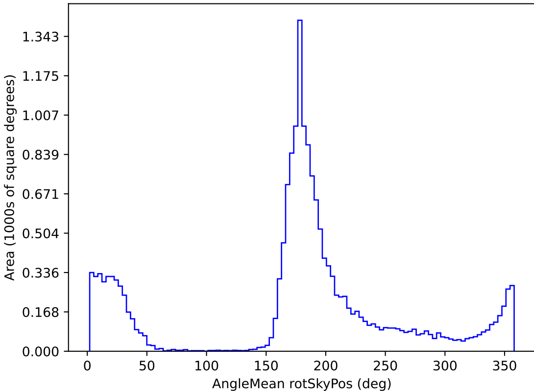
roman_v3.3_10yrs WFD g band: AngleMean rotSkyPos
