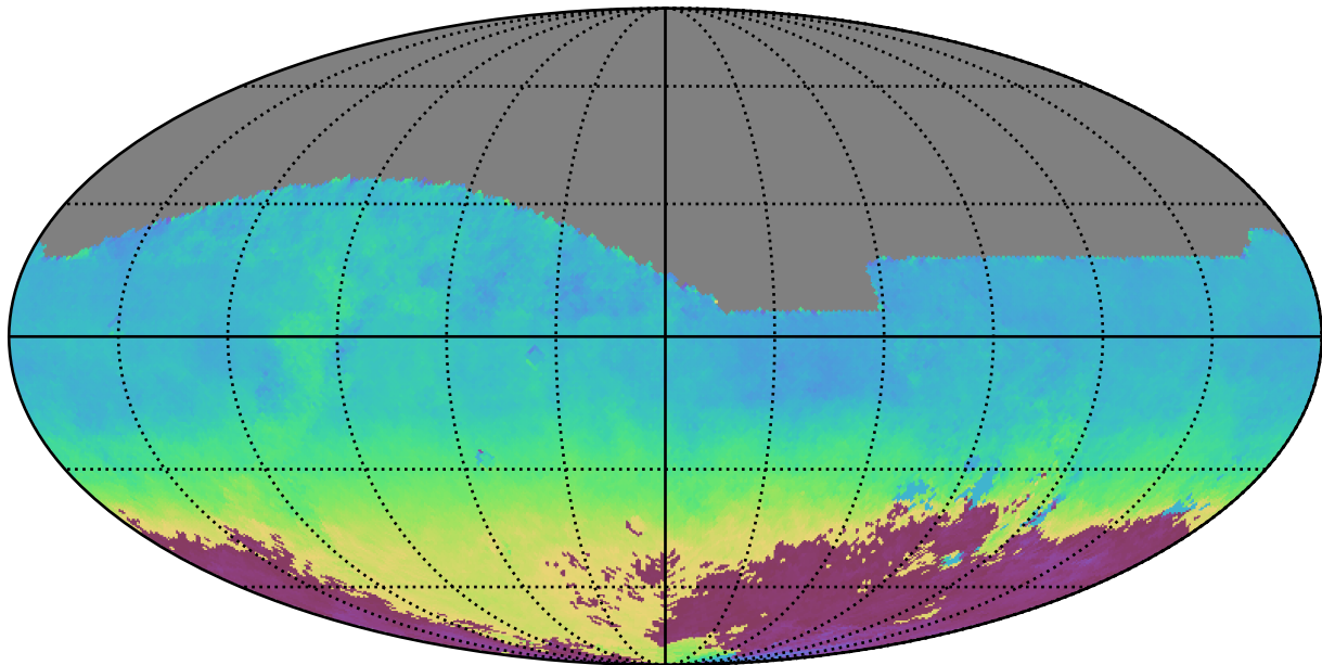
roman_v3.3_10yrs All sky z band: AngleMean rotSkyPos
