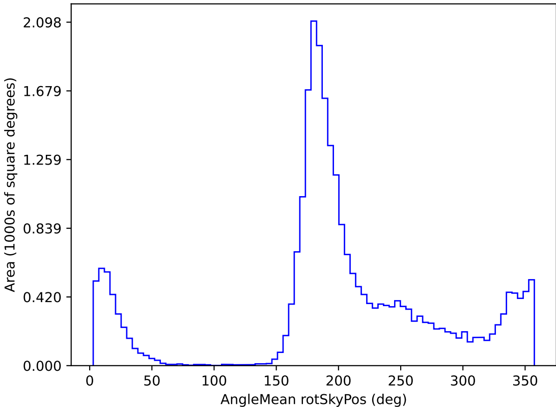
roman_v3.3_10yrs All sky z band: AngleMean rotSkyPos
