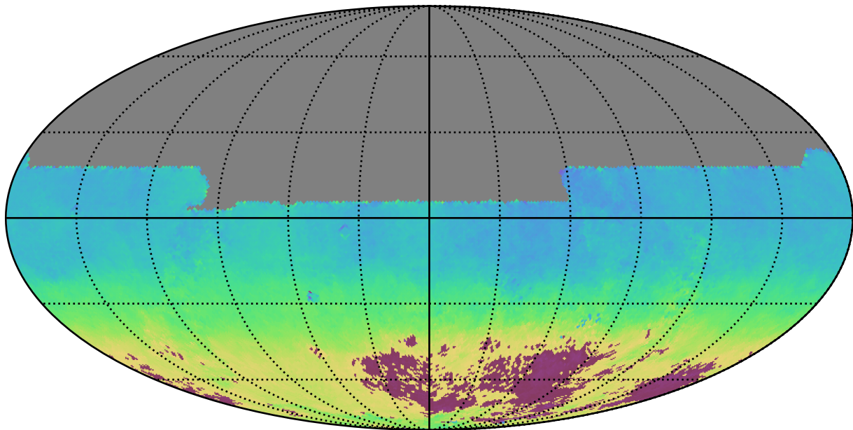
roman_v3.3_10yrs All sky y band: AngleMean rotSkyPos
