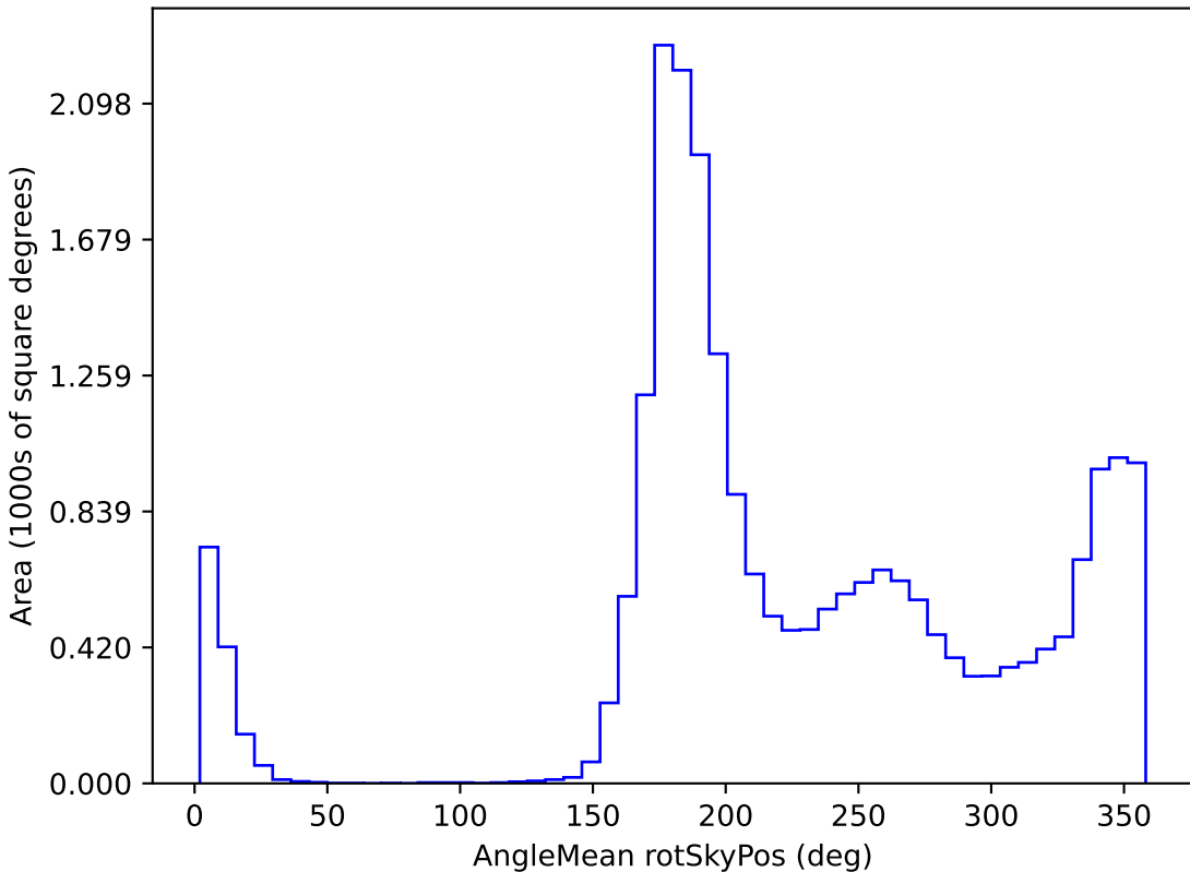
roman_v3.3_10yrs All sky y band: AngleMean rotSkyPos
