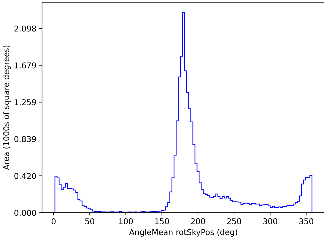
roman_v3.3_10yrs All sky r band: AngleMean rotSkyPos
