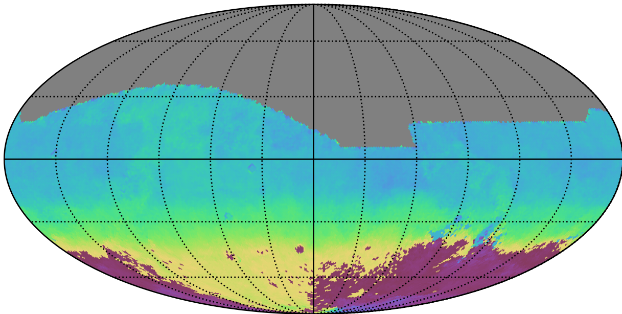
roman_v3.3_10yrs All sky i band: AngleMean rotSkyPos
