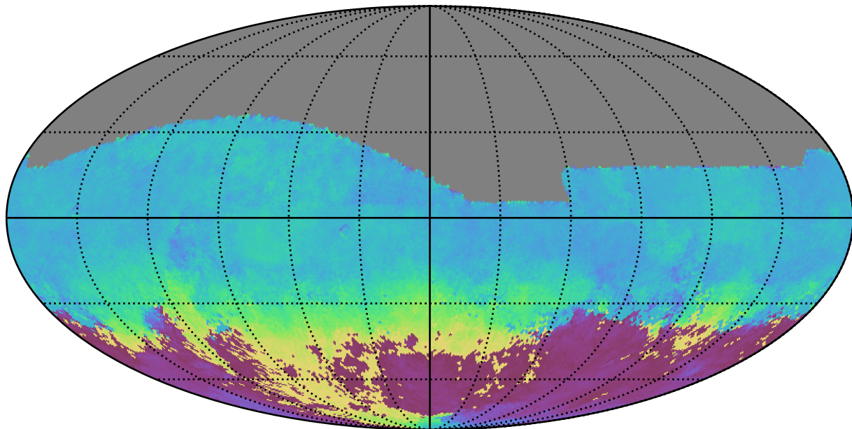
roman_v3.3_10yrs All sky g band: AngleMean rotSkyPos
