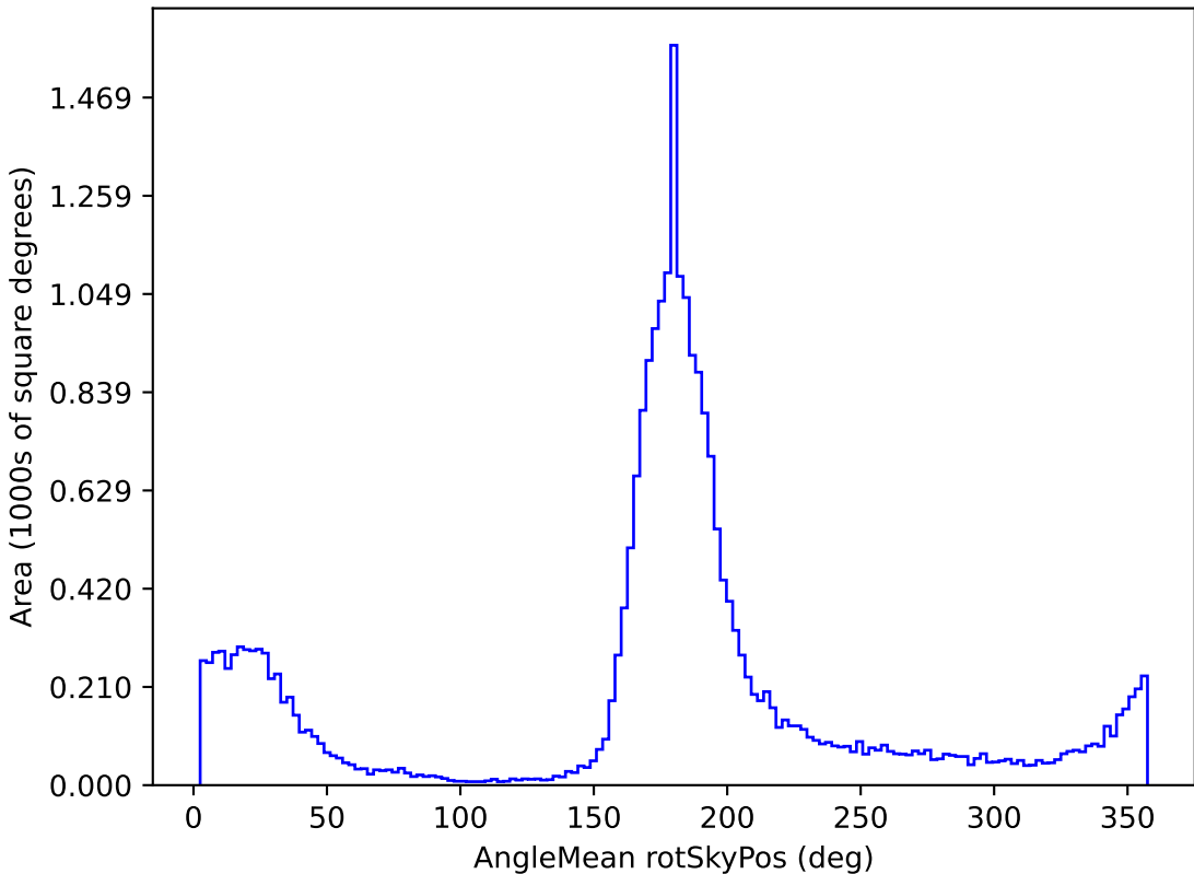
roman_v3.3_10yrs All sky g band: AngleMean rotSkyPos
