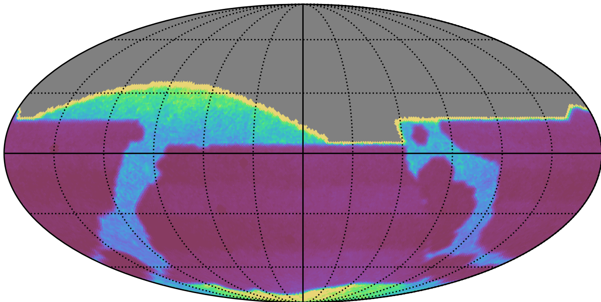
roman_v3.3_10yrs : properMotion
