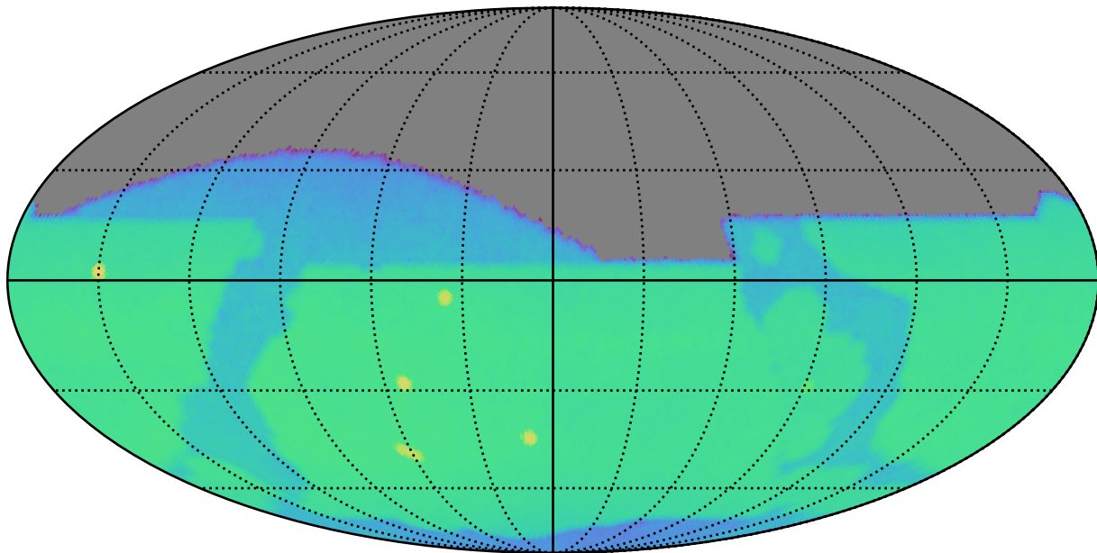
roman_v3.3_10yrs z: CoaddM5
