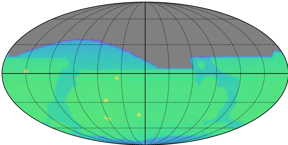
roman_v3.3_10yrs i: CoaddM5
