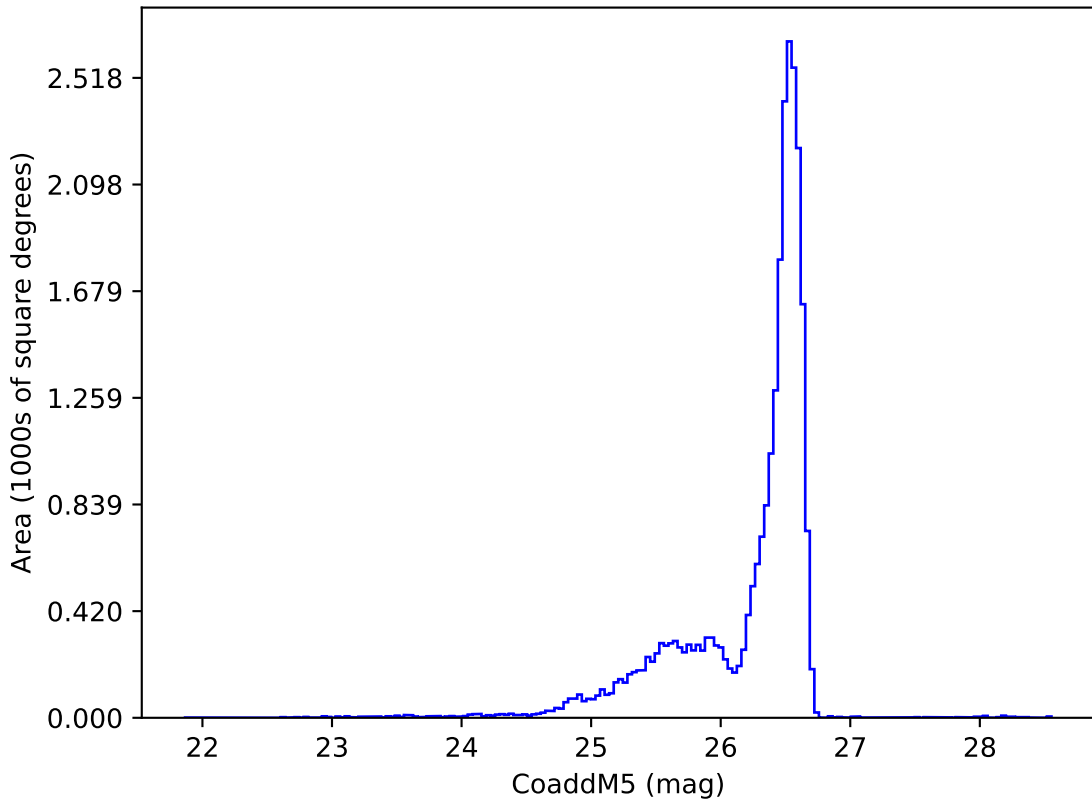
roman_v3.3_10yrs i: CoaddM5
