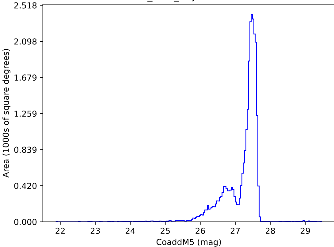
roman_v3.3_10yrs : CoaddM5
