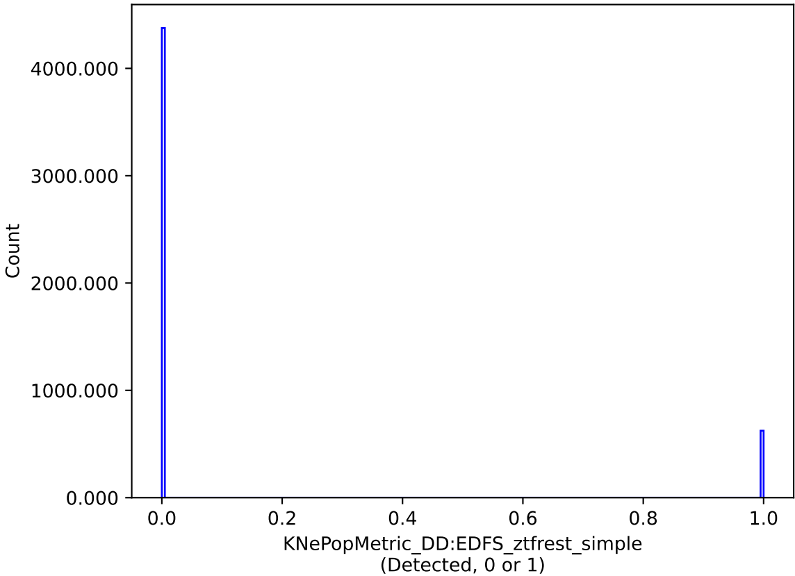
roman_v3.3_10yrs DD:EDFS: KNePopMetric_DD:EDFS_ztfrest_simple
