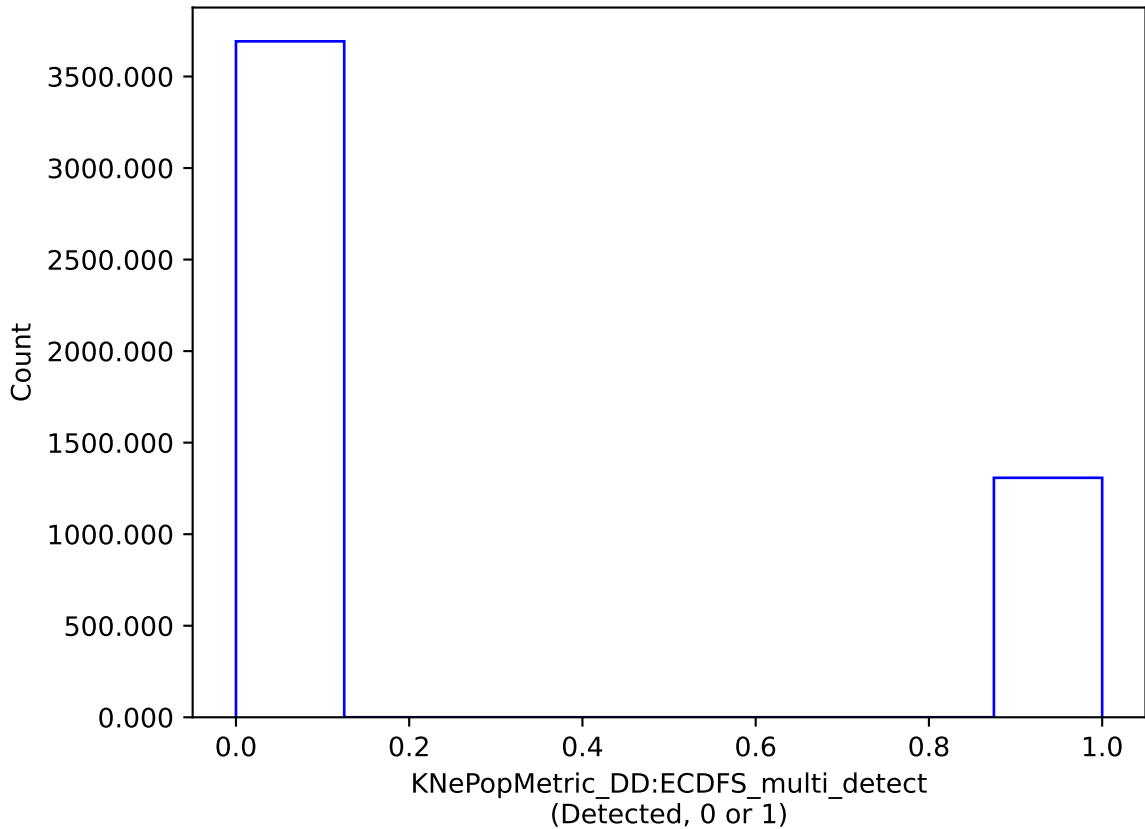
roman_v3.3_10yrs DD:ECDFS: KNePopMetric_DD:ECDFS_multi_detect
