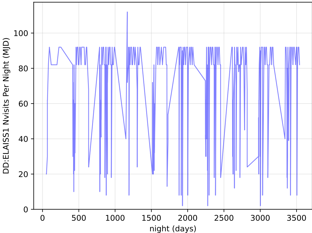
roman_v3.3_10yrs all bands: DD:ELAISS1 Nvisits Per Night
