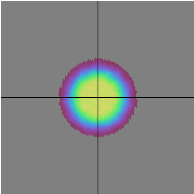
roman_v3.3_10yrs g band: DD:ELAISS1 NVisits
